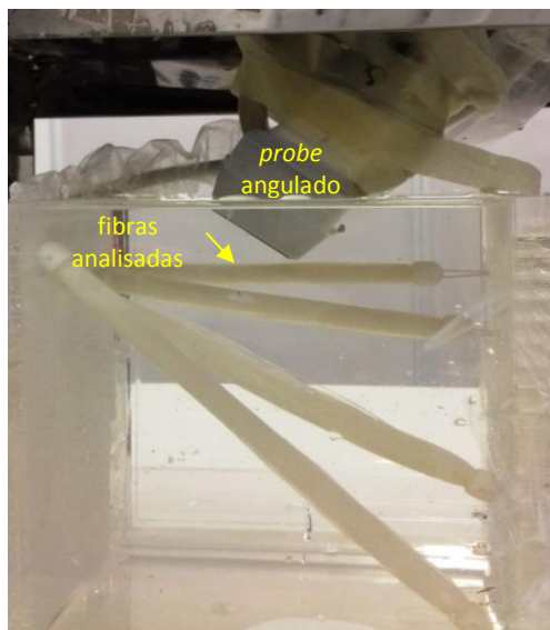
Figura 26: Fotos das aquisições (à esquerda) e imagens elastográficas (à direita) com probe nas posições A) longitudinal, B) transversal e C) oblíqua às fibras (plano x_1 - x_3 ).
