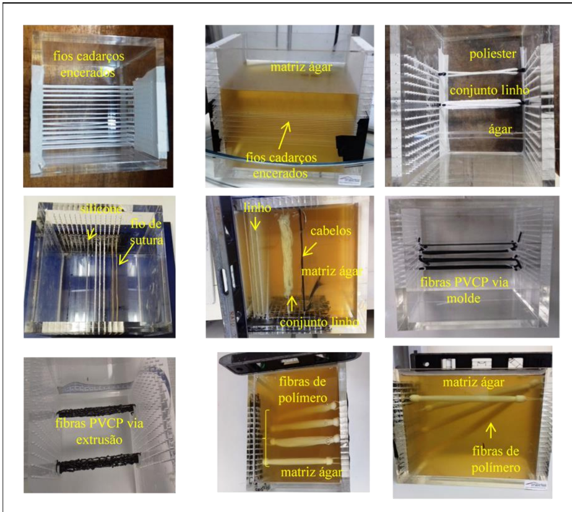
Figura 24: Disposição dos fios e fibras no molde de acrílico antes e após a imersão de ágar (Fonte: Laboratório de Ultrassom/UFRJ).
