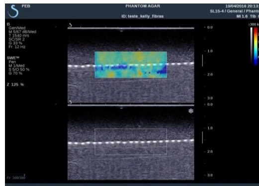
Figura 25: Posicionamento do probe paralela e perpendicularmente aos fios de nylon. À direita, observam-se as imagens elastográficas correspondentes. Note a saturação da imagem elastográfica superior, demonstrando que o módulo de Young no fio de nylon foi superior a 300 kPa no preset phantom (Fonte: Laboratório de Biomecânica PEB/COPPE/UFRJ).
