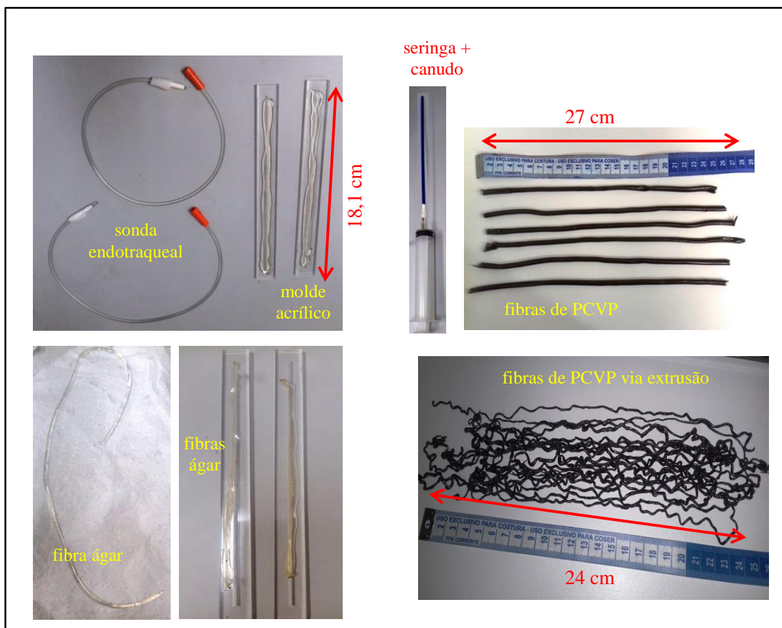
Figura 22: Fibras confeccionadas no LUS/UFRJ. À esquerda, observam-se fibras de ágar, moldadas por sonda endotraqueal e molde de acrílico. À direita, fibras de PVCP + grafite moldadas no canudo (superior) e por extrusão (inferior) (Fonte: Laboratório de Ultrassom/UFRJ).
