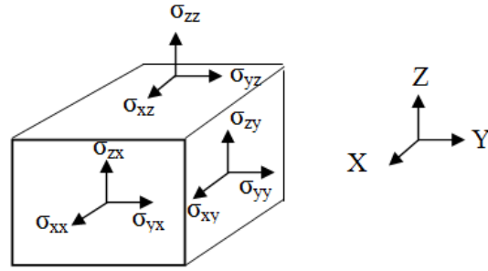
Figura 3: Ilustração de um cubo cujas faces sofrem ações de tensores tensão ( \sigma ) e deformação ( \epsilon ) nos três eixos cartesianos: X, Y e Z.
