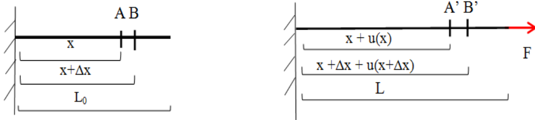
Figura 4: Ilustração do deslocamento dos pontos A e B de uma barra. Eles se deslocam pelas funções de deslocamento u(x) e u(x+\Delta x) , respectivamente, após a aplicação de uma força F .
