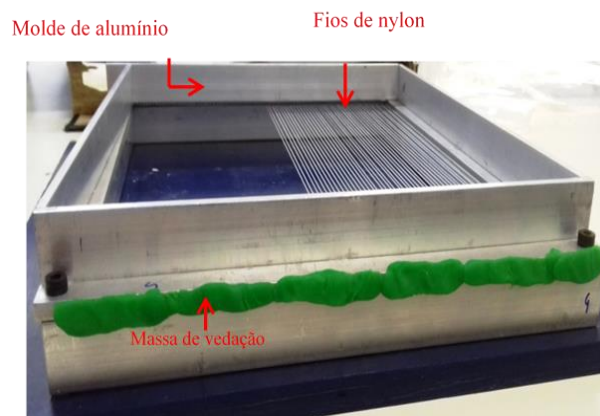
Figura 20: Molde de alumínio contendo fios de nylon (Fonte: Laboratório de Biomecânica PEB/COPPE/UFRJ e Laboratório de Opto-Mecânica da UFF).
