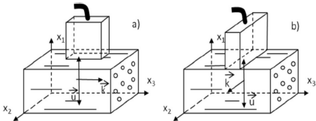
Figura 17: Esquema mostrando o probe da SSI acoplado a um sólido com fibras na direção x_3 . Na figura a), o probe está paralelo (longitudinal) às fibras e a onda de cisalhamento se propaga ( \vec{k} ) nessa direção. Na figura b), o probe está posicionado transversalmente às fibras e a onda de cisalhamento se propaga nessa direção. Em ambas as ilustrações, o deslocamento das partículas ( \vec{u} ) é perpendicular a x_3 . (Figura retirada do artigo de ROYER et al. (2011); sob permissão da Copyright Clearance Center's RightsLink ®).
