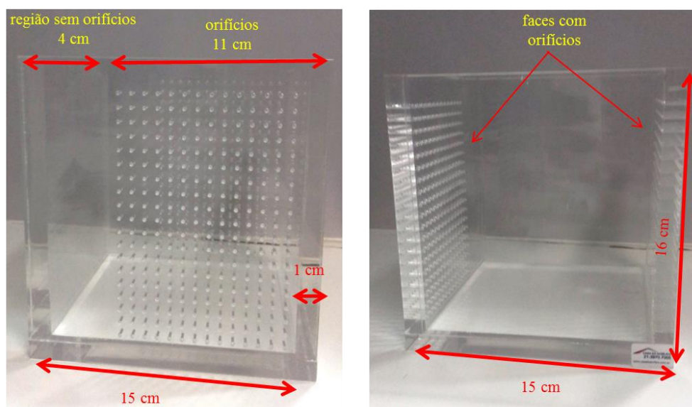
Figura 21: Molde de acrílico e suas dimensões (Fonte: Laboratório de Biomecânica PEB/COPPE/UFRJ).
