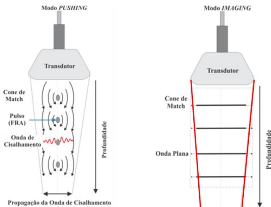
Figura 11: Esquema da elastografia SSI no modo pushing (à esquerda) e modo imaging (à direita). A frente da onda quase plana é representada em vermelho à direita da figura. FRA: força de radiação acústica.
