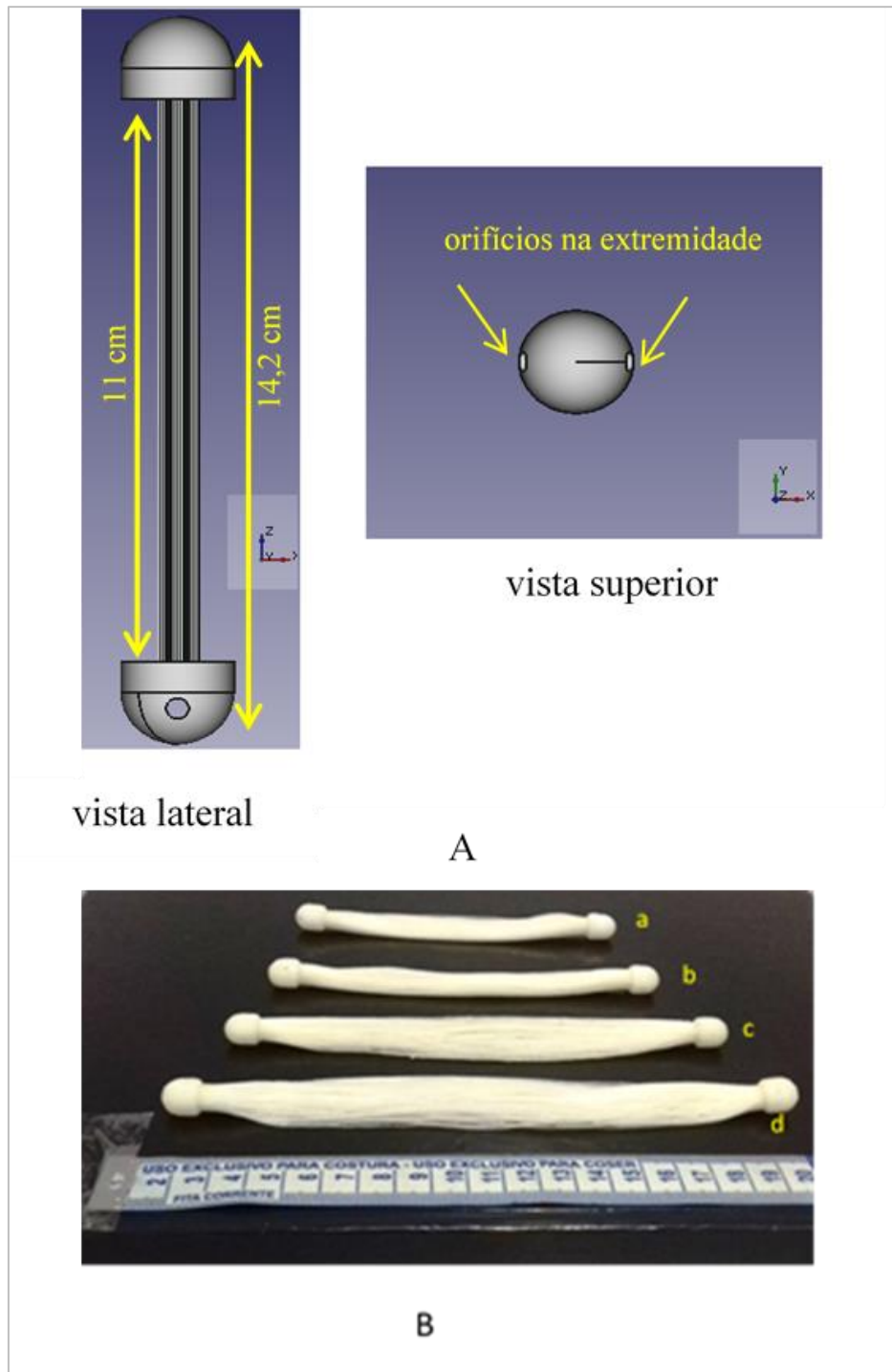
Figura 23: A) Projeto do conjunto de fibras de comprimento 14,2 cm, numa vista lateral e superior. B) quatro conjuntos de fibras produzidas pela impressora 3D, cujos comprimentos são: a = 13 cm, b = 14,2 cm, c = 17 cm e d = 19,3 cm.
