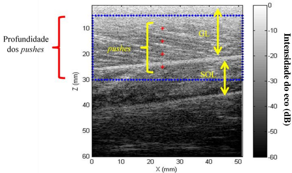
Figura 12: Imagem modo-B gerada pelo equipamento homemade ultrafast ultrasound scanner . Os asteriscos vermelhos representam a profundidade dos quatro pushes nos músculos gastrocnêmio lateral (GL) e sóleo (SL). A profundidade da imagem é 60 mm e a largura, 50 mm.
