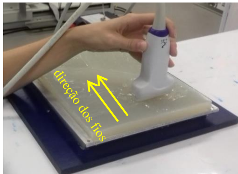
Figura 25: Posicionamento do probe paralela e perpendicularmente aos fios de nylon. À direita, observam-se as imagens elastográficas correspondentes. Note a saturação da imagem elastográfica superior, demonstrando que o módulo de Young no fio de nylon foi superior a 300 kPa no preset phantom (Fonte: Laboratório de Biomecânica PEB/COPPE/UFRJ).
