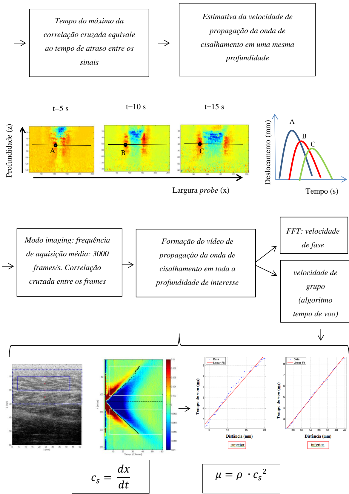
Figura 16: Diagrama de blocos contendo uma simplificação do processamento de sinais para aquisição dos dados do módulo de cisalhamento da elastografia SSI. FFT: fast Fourier transform (transformada rápida de Fourier ).
